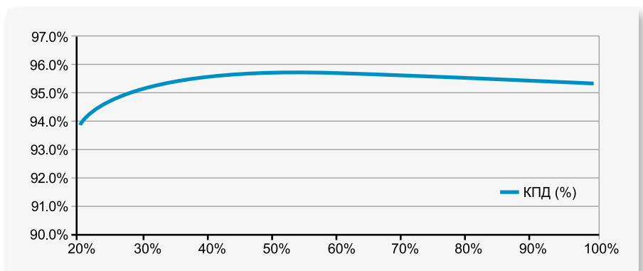
Liebert® NX — график КПД
